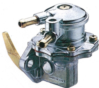
Versione "N" Izvedba "N"
